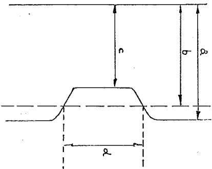
Fig. 1. Dimensies van een lasverbinding van afdichtingsfolies.
